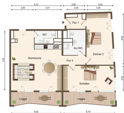
Grundriss_KBN_355.jpg
