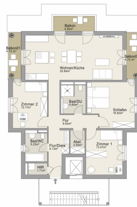
Grundriss 1OG Zus
